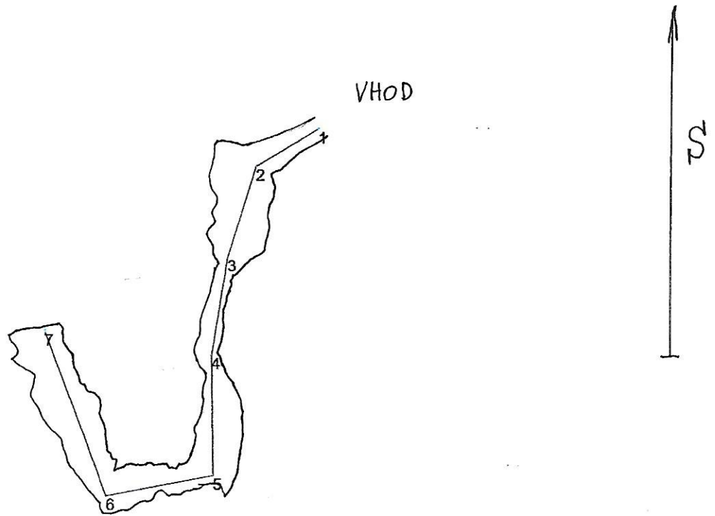
Iztegnjen profil
